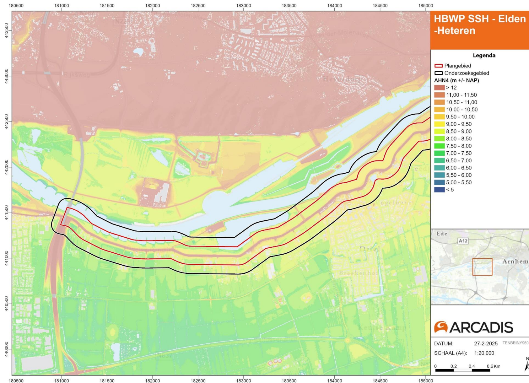
Figuur P-1: Uitsnede van Figuur P voor het westelijk deel van het onderzoeksgebied.
